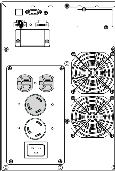
Рисунок 50. Модель PW9130G3000T-XL
