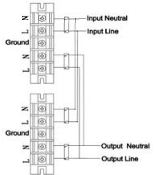
Рис. 12: Подключение кабеля питания
