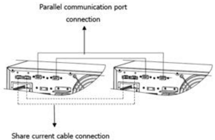
Рис. 13: Схемы соединений для моделей ИБП в корпусах типа Rack
