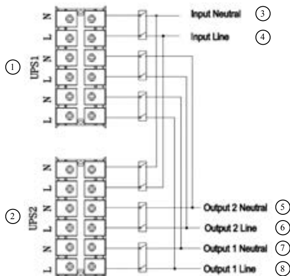
Рис. 10: Подключение кабеля питания
